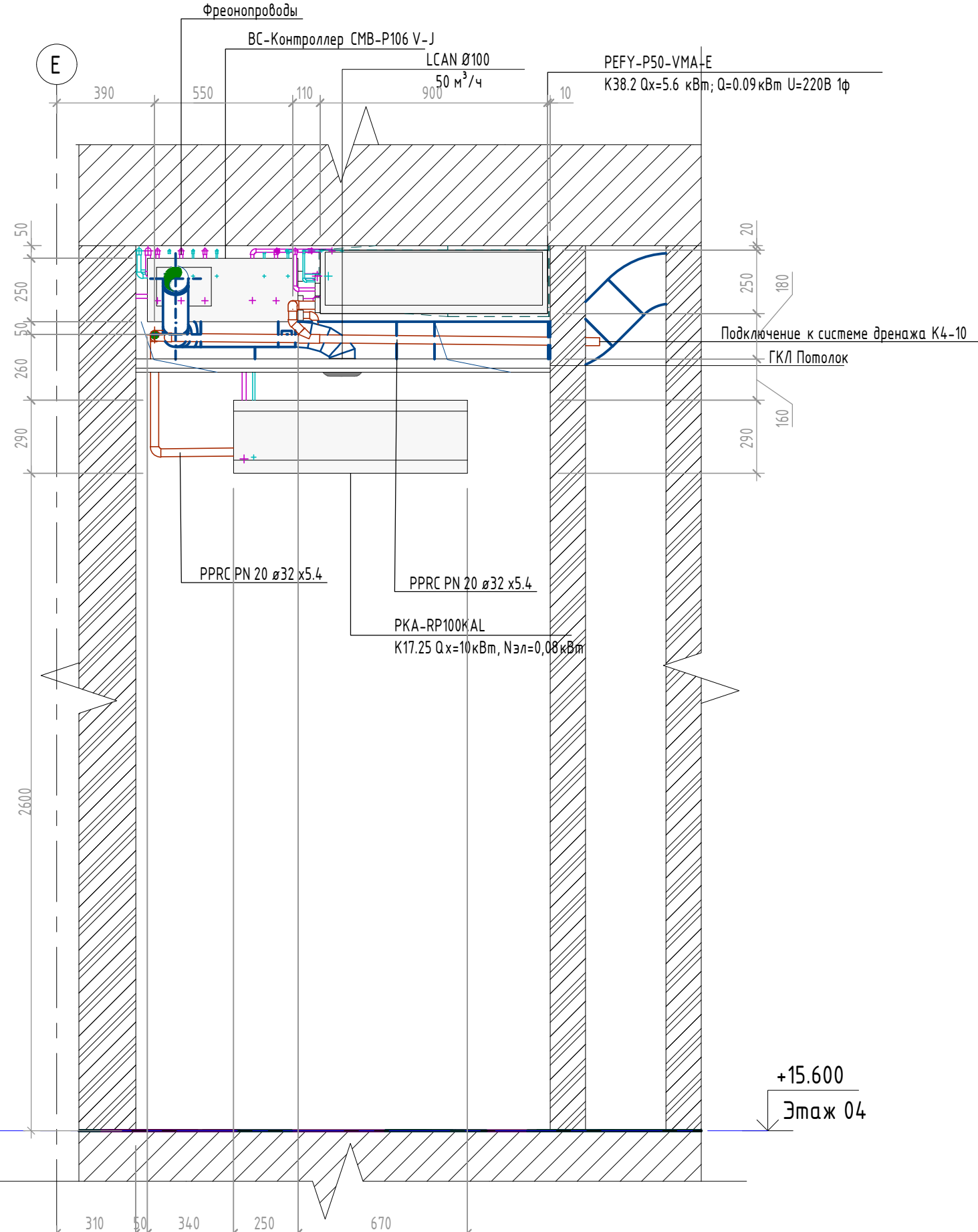
РАЗРЕЗ 8-8. М1:20
