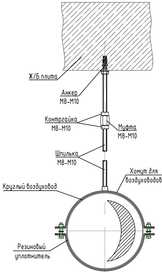
Элементы крепления воздуховодов к ЖБ плите
