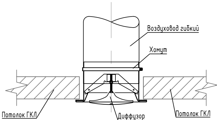
Узел крепления диффузора в потолке ГКЛ
