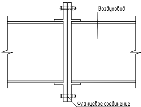
Участок соединения воздуховодов
