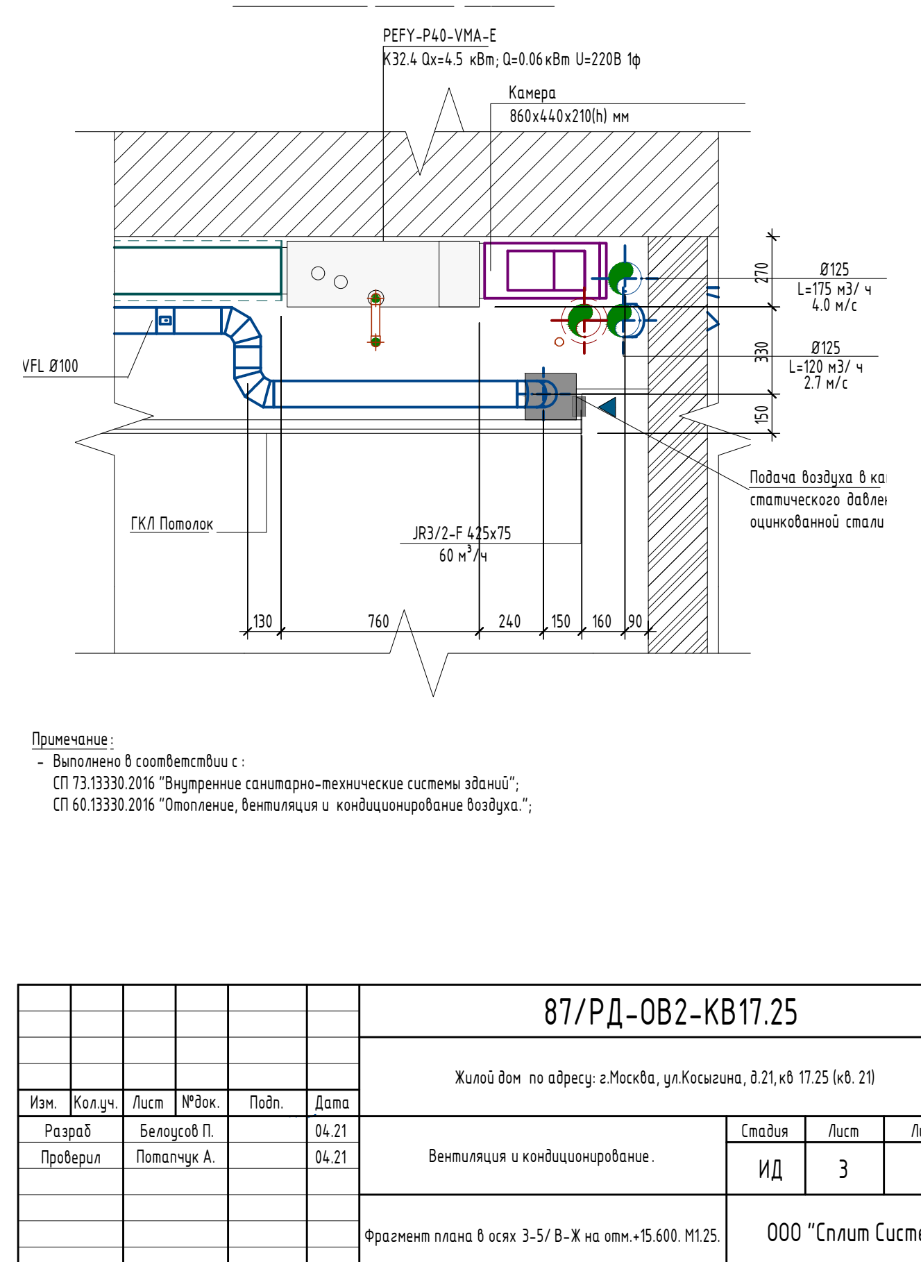
PA3PE3 3-3. M1:20
