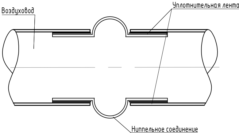
Участок соединения воздуховодов
